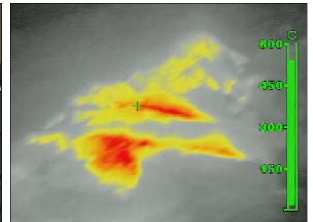
Originalbild des Brandherdes, aufgenommen mit der Wärmebildkamera des Unterabschnittes Pottendorf - deutlich über 500°C! ↑
